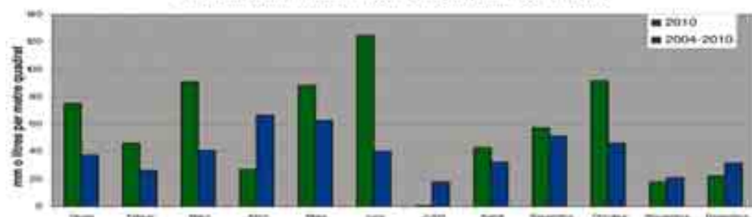
Precipitacions a l'Observatori de Pujalt (Alta Anoia - 750m)
